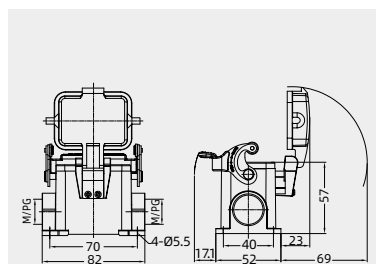
1) : Structure 1 ( *M/PG=M25/PG16 Using Structure 1)
